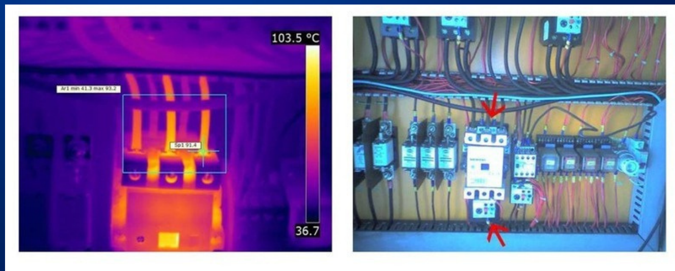
Exemplo de foto digital e respectivo termograma
